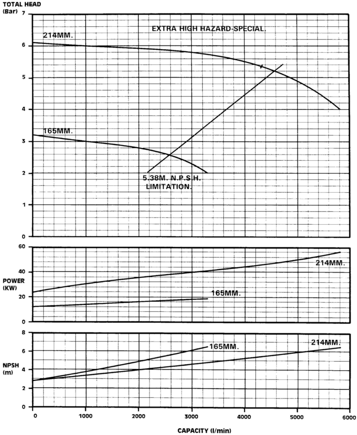
شكل (ب/2-11أ) المضخات للخطورة العالية حسب LPC
